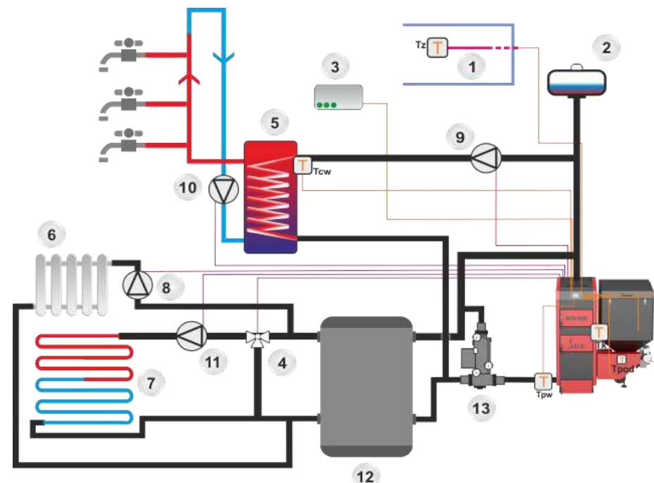
Rysunek 14.4 Podłączenie kotła do instalacji grzewczej z laddomatem i buforem
