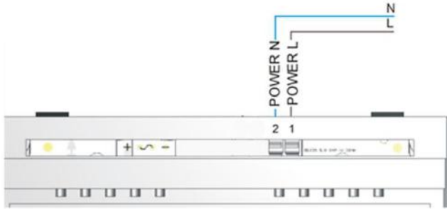
Rys. 6.9 Podłączenie zasilania sieciowego do ecoLAMBDA 2B
