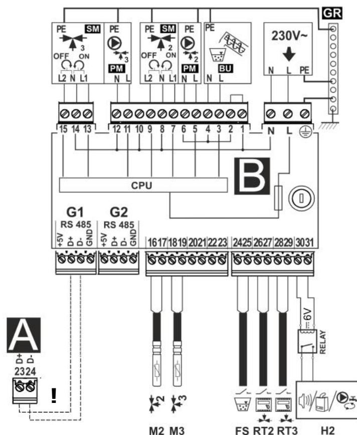
Schemat połączenia elektrycznego – dodatkowy moduł B: M2 – czujnik temperatury mieszacza 2 typu CT4, M3 – czujnik temperatury mieszacza 3 typu CT4, RT2 – standardowy termostat pokojowy mieszacza 2, RT3 – standardowy termostat pokojowy mieszacza 3, FS – czujnik poziomu paliwa do obsługi podajnika BU, H2 – wyjście napięciowe do sterowania kotłem rezerwowym, sygnalizacją alarmów oraz pompą cyrkulacji, RELAY – przekaźnik 6 VDC, L N PE – zasilanie 230V~, PM3, PM4 – pompa mieszacza 3 i 4, SM3, SM4 – siłownik mieszacza 3 i 4, BU – podajnik paliwa z bunkra do zasobnika kotła, CPU – sterowanie, A – moduł A regulatora, ! – łączyć wyłącznie dwuprzewodowo (połączenie czteroprzewodowe może uszkodzić regulator).
