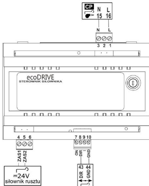
Schemat połączenia elektrycznego modułu ecoDRIVE (sterownik siłownika).
